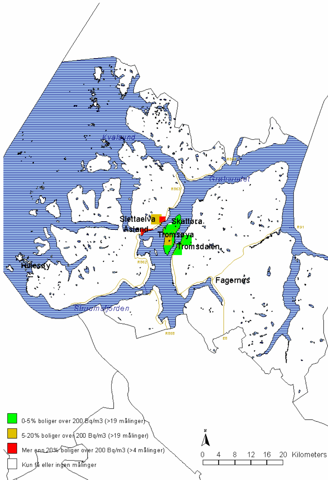
Figur 1: Områdekart for Tromsø kommune. Oversikt over måleresultater fra "Radon 2000/2001", der radonkonsentrasjonen i inneluft ble målt i 2 % av boligmassen i kommunen.
