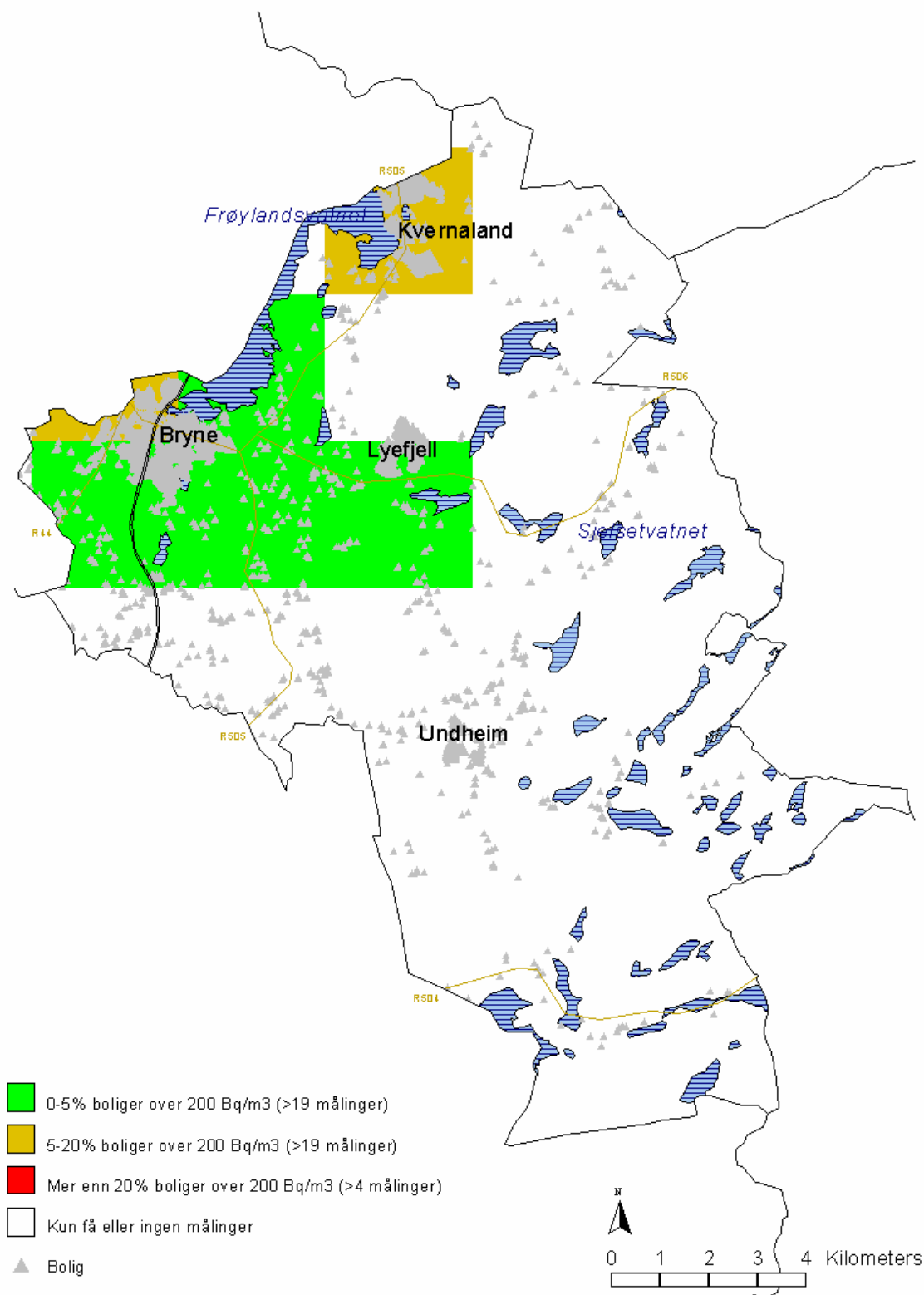
Figur 1: Områdekart for Time kommune. Oversikt over måleresultater fra "Radon 2000/2001", der radonkonsentrasjonen i inneluft ble målt i 10 % av boligmassen i kommunen.
