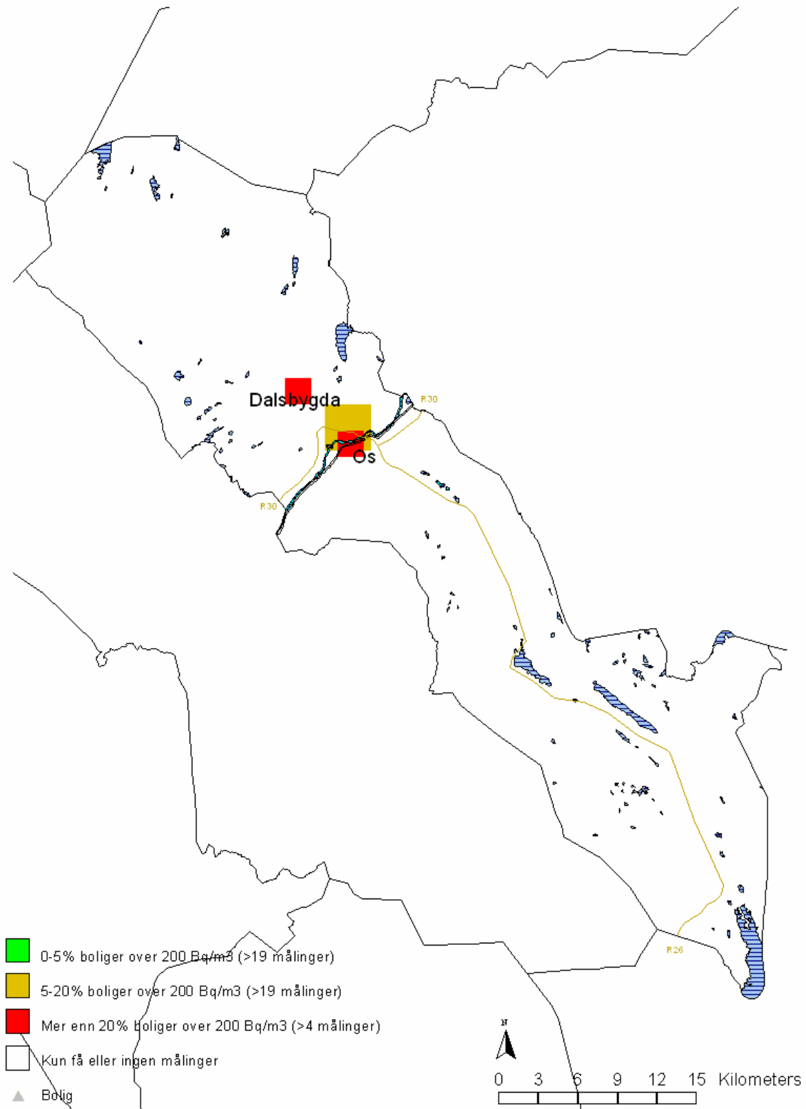
Figur 1: Områdekart for Os kommune. Oversikt over måleresultater fra "Radon 2000/2001", der radonkonsentrasjonen i inneluft ble målt i 9 % av boligmassen i kommunen
