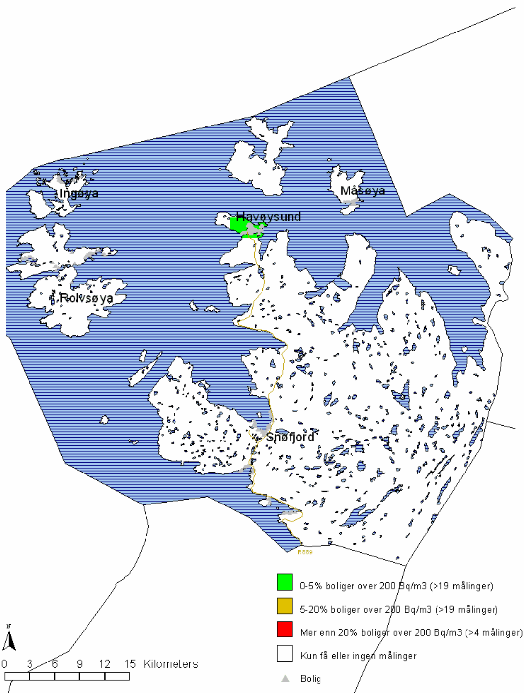
Figur 1: Områdekart for Måsøy kommune. Oversikt over måleresultater fra "Radon 2000/2001", der radonkonsentrasjonen i inneluft ble målt i 14 % av boligmassen i kommunen.
