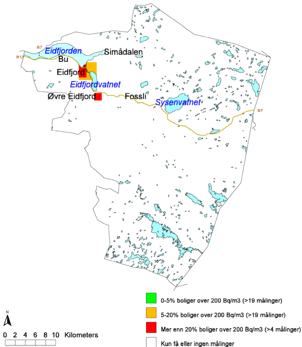
Figur 1: Områdekart for Eidfjord kommune, basert på målinger i forbindelse med prosjektet RaMAP. Kartet er utarbeidet på grunnlag av 90 målinger.
